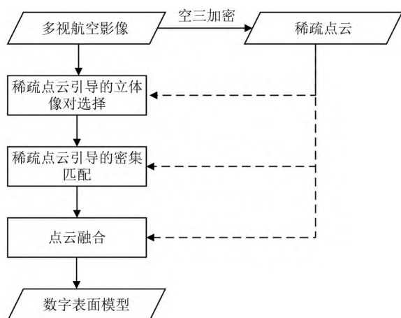
图1 稀疏点云引导的航空影像DSM生成流程图
